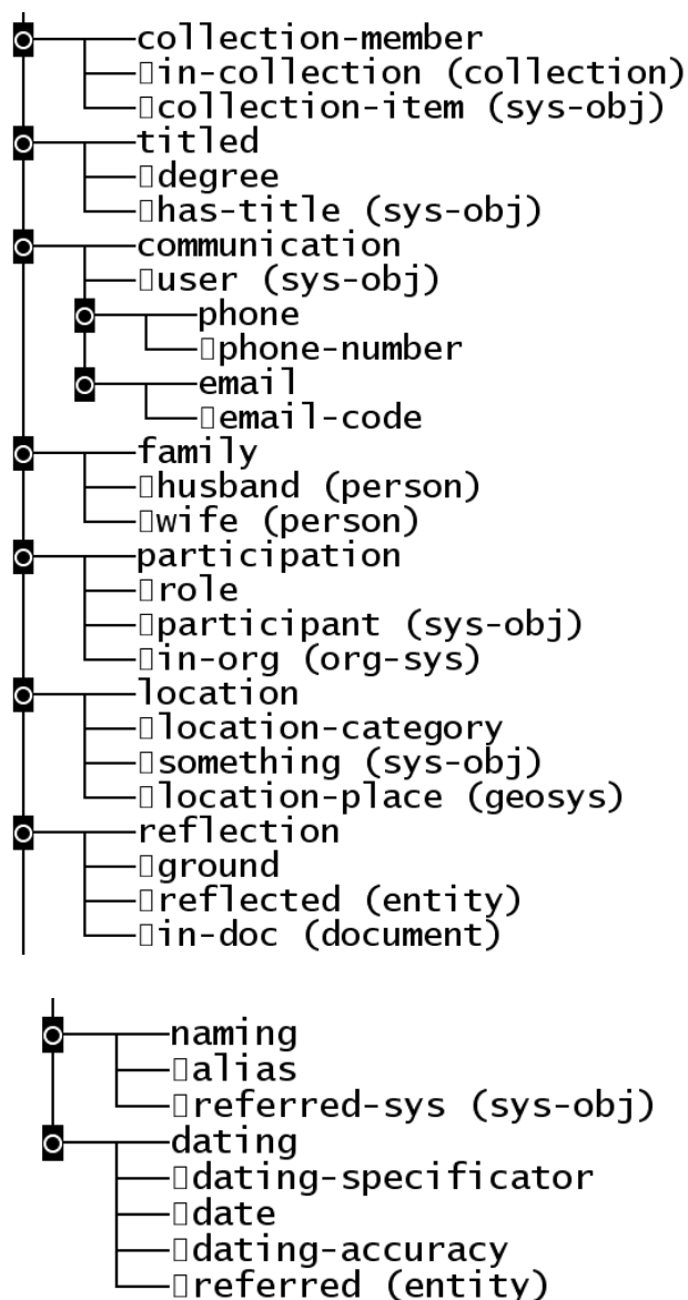
Рис. 5. Основные классы и отношения онтологии неспецифических сущностей
